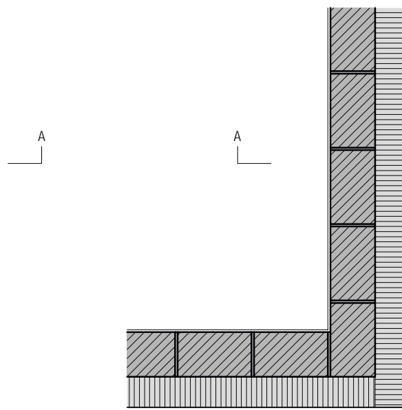
Grundriss 2. Schicht
