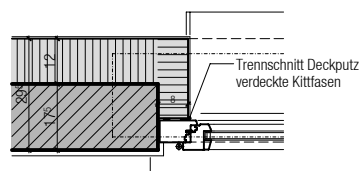
Grundriss Leibung
