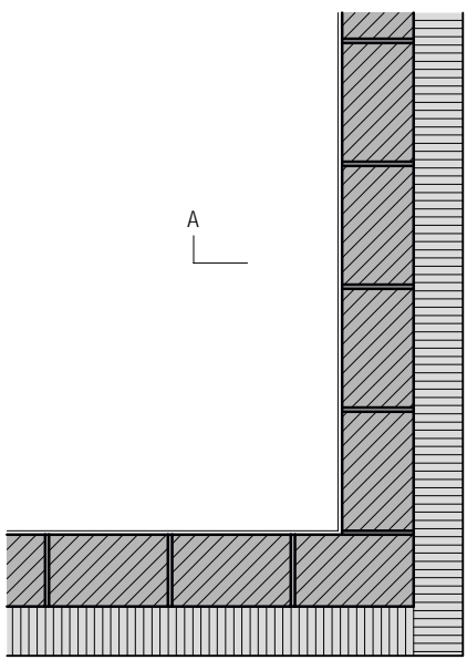
Grundriss 1. Schicht
